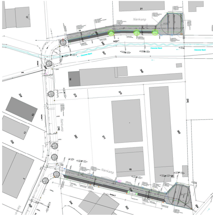
Bild: Lageplan Straßenendausbau
