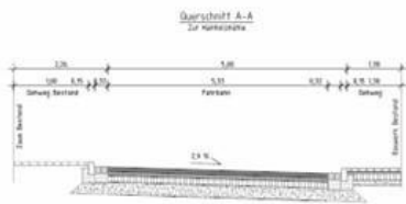
Bild: Übersichtslageplan Verkehrsanlagen mit Querprofil und Ausschnitt der Einzugsgebiete des Entwässerungsplanes
