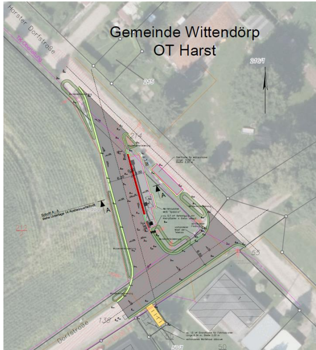
Abbildung 1 Bushaltestelle und Wendeanlage Harst
