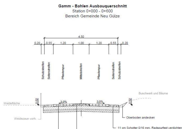
Bild 2: Genehmigungsplanung Ausbauquerschnitt
